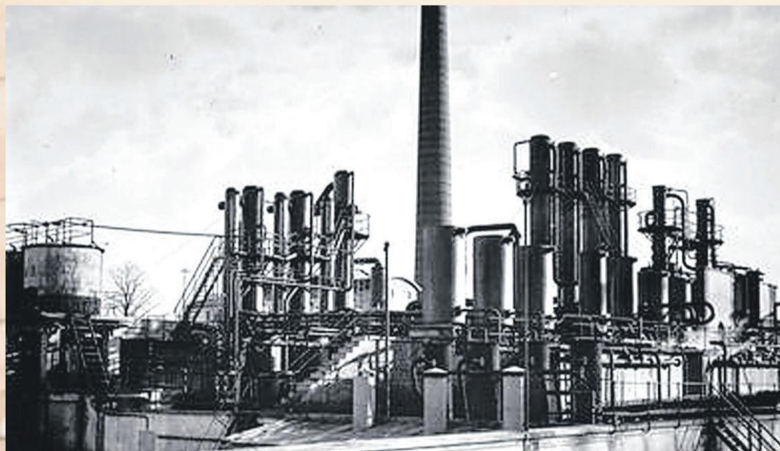
Rafineria w Libuszy urządzenia destylacyjne
