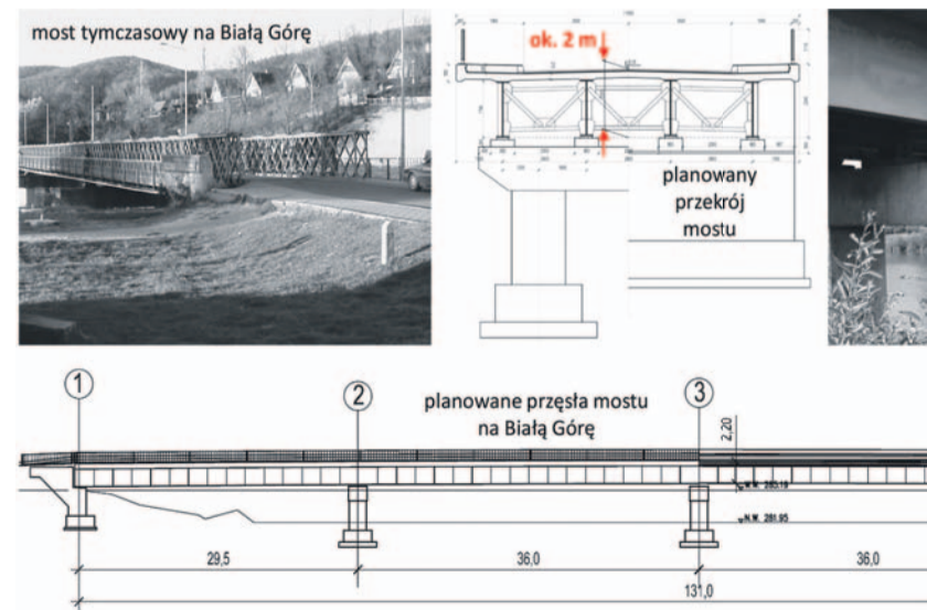
Rys. 2. Most na Sanie w Iskanie. Taka sama konstrukcja miała być w 1990 roku zbudowana
