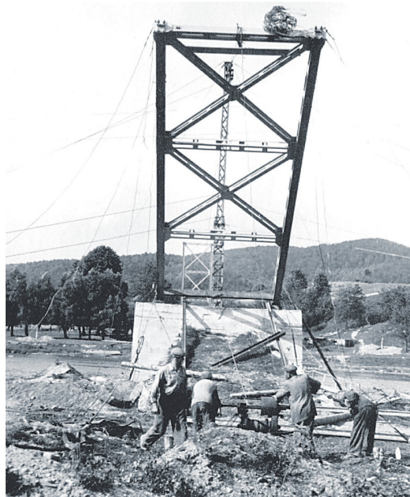
ab Budowa kładki wiszącej na Białą Górę. Czas powstania: 1958 r.
