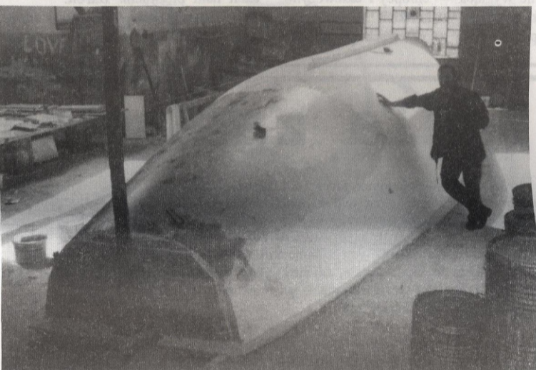
Pełnomorski jacht budowany przez J. Jagodę.
