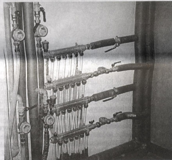
Platanina rur, rurek i zaworków – tak wygląda znajdująca się na klatce schodowej instalacja, dzięki której każde z mieszkań jest całkowicie opomiarowane. Niebawem zniknie ona pod estetyczną boazerią.
