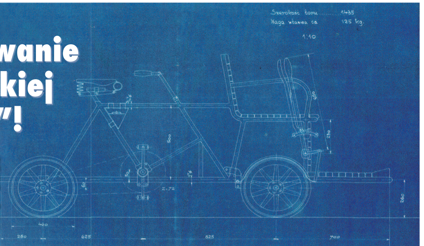
Rysunek techniczny nr 15184 przedstawiający drewnianą dźwignię dla popędu nożnego z dwoma siedzeniami i z ławką na przodzie, 1925 r.
